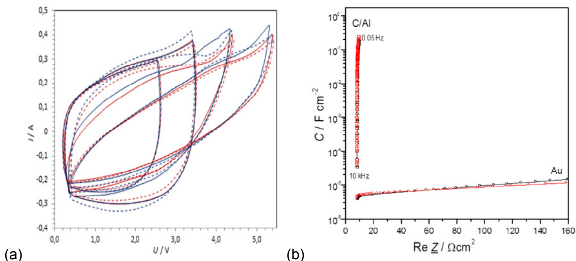
Abbildung 20: (a) Cyclovoltogramme von quartären Ammoniumsalzen in Acetonitril an Aktivkohle-Aluminium-Elektroden ( 6,25\ cm^2 ). Spannungsvorschub 100\ mV\ s^{-1} . — — — wasserhaltiges Et_3MeNBF_4 , — — — Et_4NBF_4 — — — wasserfrei, — — — wasserfrei stabilisiert. Elektrolytwiderstand ( R_e \approx 1,5\ \Omega ) korrigiert. (b) Impedanzspektren: gewöhnlicher (—) und stabilisierter (—) Elektrolyt an glatten Goldelektroden (geringe Kapazität) und porösen Kohlenstoffelektroden (hohe Kapazität), geringer Widerstand.
