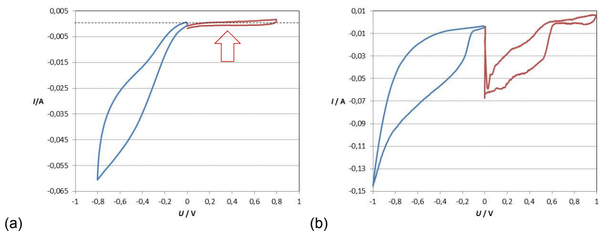
Abbildung 16: (a) Cyclovoltogramm einer Zelle aus \text{RuO}_2 -Elektrode (aus \text{RuCl}_3 , 380 °C, 2 h, \sim 0,4 \text{ mg cm}^{-2} ) und kommerzieller Aktivkohle-Gegenelektrode in Kaliumchloridlösung, 2. Zyklus, 5 \text{ mV s}^{-1} . Pfeil: Lade-Entlade-Zyklus über das Spannungsfenster. (b) Zum Vergleich: laserbehandeltes \text{RuCl}_3 .
