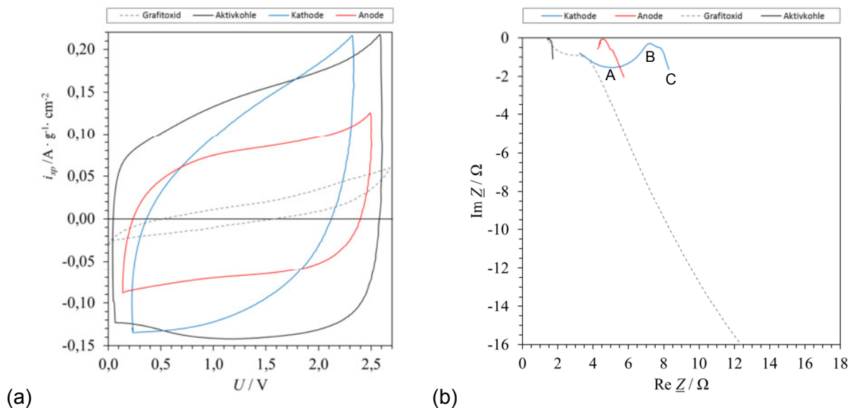
Abbildung 9: (a) Strom-Spannungskurven (CV) von anodisch und kathodisch formierter Aktivkohle (6-molare Kalilauge, 6,5 \text{ V} ; \sim 170 \text{ mA cm}^{-2} , 6902 \text{ As} ). Zweielektroden-Anordnung mit frischer Aktivkohle-Gegenelektrode, 1 \text{ M Et}_4\text{NBF}_4 in Acetonitril; 20 \text{ mV s}^{-1} ; IR-Drop korrigiert: Aktivkohle ( 1,46 \text{ }\Omega ), Anode nach Elektrolyse ( 4,45 \text{ }\Omega ), Kathode ( 4,91 \text{ }\Omega ), PTFE- und rußgebundenes Graphitoxid auf Alufolie ( 1,9 \text{ }\Omega ). Elektrodenquerschnitt 6,25 \text{ cm}^2 . (b) Impedanzspektren: A Kontaktwiderstand Aktivschicht/Träger, B Aktivschicht/Elektrolyt: Korngrenzen- und Durchtrittswiderstand, C poröse Elektrode: Diffusionsimpedanz.
