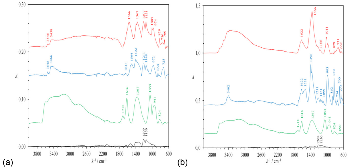
Abbildung 8: FTIR-Spektren von Aktivkohleelektroden nach anodischer (rot) bzw. kathodischer Formierung (blau) in 6-molarer Kalilauge: (a) nach 6902 As ( 0,17 \text{ A cm}^{-2} , 6,5 \text{ V} ), (b) nach 7300 As, im Vergleich zum Ausgangszustand (schwarz) und Grafitoxid (grün) als Modellschicht: \sim 3400 \text{ cm}^{-1} \nu(\text{OH}) , 1719 \text{ cm}^{-1} \nu(\text{C=O}) , 1614 \text{ cm}^{-1} \nu(\text{C=C}) , 1360 \text{ cm}^{-1} \delta(\text{C-OH}) , 1047 \text{ cm}^{-1} \nu(\text{C-O}) , 924 \text{ cm}^{-1} \nu(\text{C-O-C}) in Epoxid.
