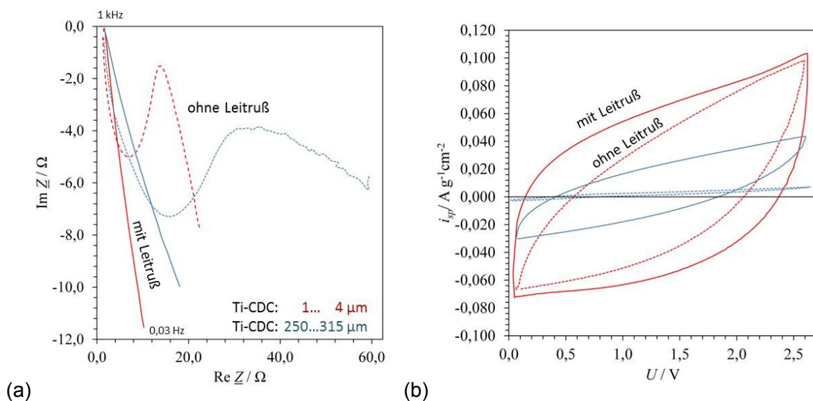
Abbildung 4: Vergleich zweier Ti-CDC-Elektroden mit unterschiedlichen Partikelgroen ohne und mit 5 % Leitrufzusatz: (a) Impedanzspektrum, (b) voltammetrische Lade-Entlade-Kurve in 1 \text{ mol L}^{-1} \text{ Et}_4\text{NBF}_4 in Acetonitril.
