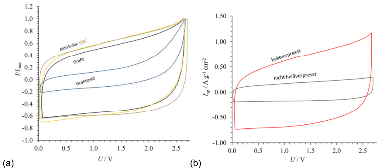
Abbildung 11: (a) Voltammetrische Strom-Spannungskurven, auf den größten Strom bezogen: Aktivkohle/SBR-NaCMC, CDC-Material/SBR-NaCMC, Grafit/PTFE, Grafitoxid/SBR-NaCMC. Zweielektroden-Anordnung, 50 mV/s, 1 M Et 4 NBF 4 in Acetonitril, I/R -Drop korrigiert, Elektrodenquerschnitt 6,25 cm 2 . (b) Aktivkohle (Kuraray YP 50F + 5 % Ruß C65 + 2 % NaCMC + 3 % SBR) auf mit Leitgraphit grundierter Aluminiumfolie mit Heißverpressung (170 kN, 120 °C, 10 s).
