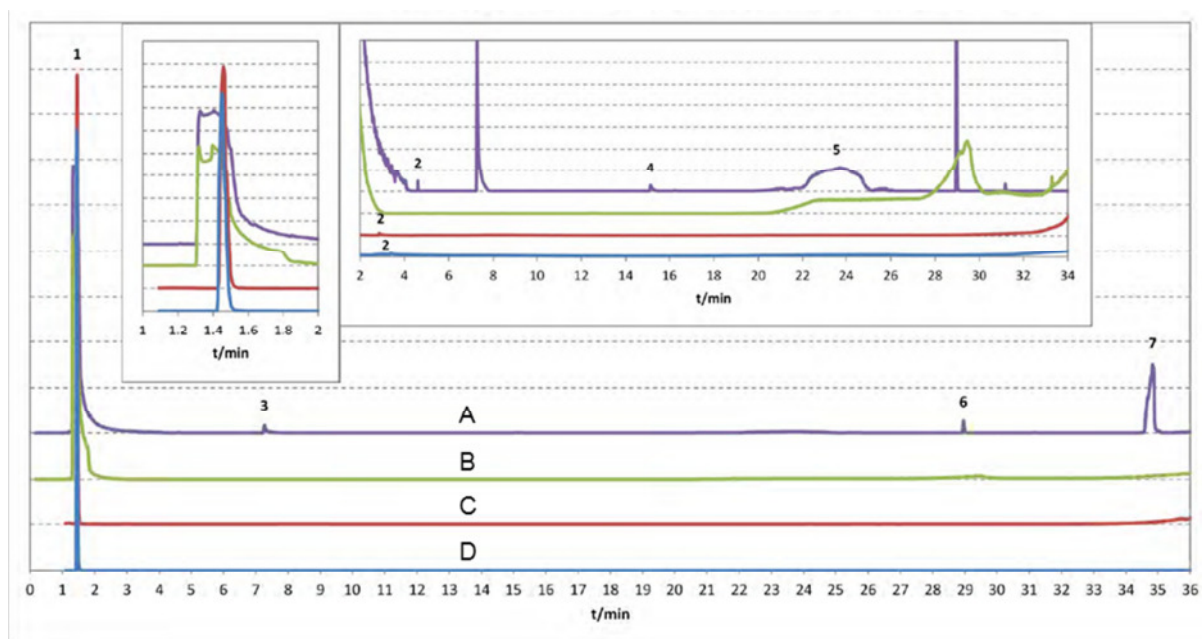
Abbildung 18: Gaschromatogramme von bei 90 °C über 76 Tage thermisch gealterten Elektrolytlösungen: A Et_4NBF_4 in trockenem Acetonitril, stabilisiert; B Et_4NBF_4 in trockenem Acetonitril, unstabilisiert (Honeywell). Frische Vergleichsproben: C 1 mol L -1 Et_4NBF_4 , D 1 mol L -1 Et_3(CH_3)NBF_4 in Acetonitril. Peaks: 1 Acetonitril (Säulentemperatur 60 °C), 2 Cyclohexanon (A, 68 °C), Acetamid (B), 3 Isocyanatocyclohexan (81 °C), 4 N -Cyclohexylformamid (121 °C), 5 Triethylamin (172 °C), 6 Dicyclohexylcarbodiimid (179 °C), 7 1,3-Dicyclohexylharnstoff (238 °C).
