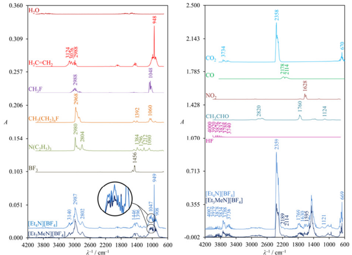
Abbildung 17: TGA-IR-Messungen an quartären Ammoniumsalzen unter Stickstoff (links) und Luftatmosphäre (rechts). IR-Spektren und Referenzspektren.
