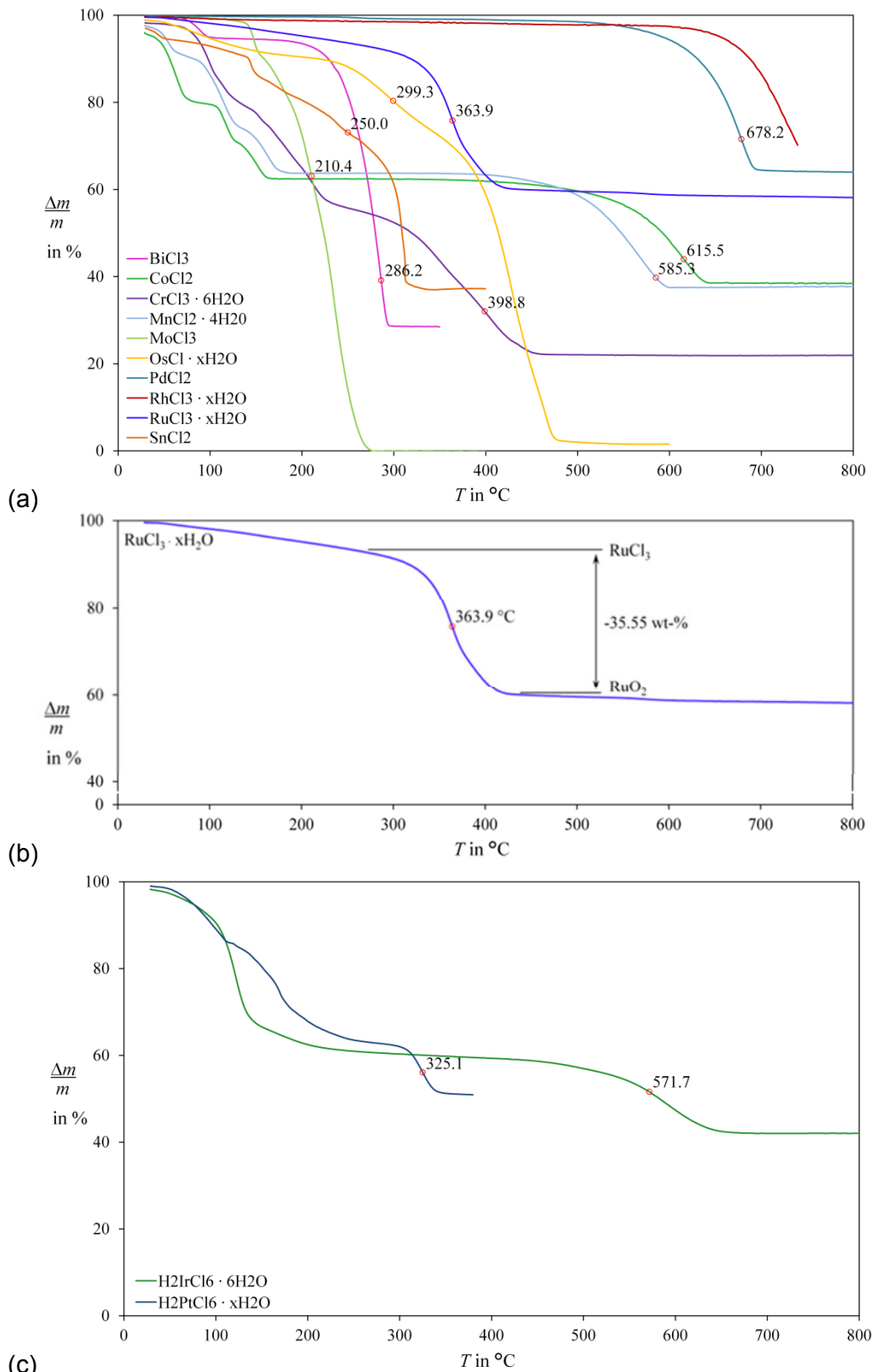
Abbildung 13: (a) Thermogravimetrische Analyse von Metallchloriden: Umwandlungstemperaturen in die Oxide (in °C). (b) wasserhaltiges Rutheniumtrichlorid. (c) Hexachloridoiridiumsäure und Hexachloridoplatinsäure.
