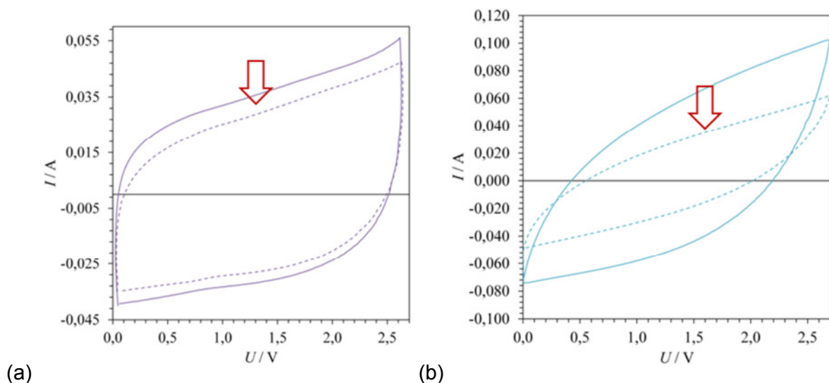
Abbildung 7: Alterung von Ti-CDC-Elektroden mit unterschiedlichen Bindern im Verlauf von 100 Lade-Entlade-Zyklen (Pfeil): Zweielektrodenanordnung, Elektrolyt: 1 mol \text{L}^{-1} \text{Et}_4\text{NBF}_4 in Acetonitril, 50 \text{ mV s}^{-1} : (a) 1-4 \mu\text{m} Ti-CDC + 5 % Vulcan XC72R + 2 % Na-CMC + 3 % SBR; Degradation 21 %; (b) 85 % Ti-CDC + 5 % Vulcan XC72R + 10 % PTFE, Degradation 47 %.
