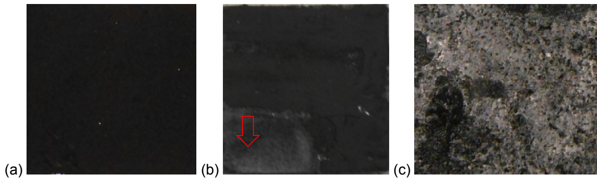
Abbildung 1: (a) Stabile Beschichtung: Ti-CDC + 5–10 % PTFE-Suspension + \leq 5 % Ruß Vulcan XC 72R, 60 °C. (b) Mechanische Ablösung: Ti-CDC + 3 % SBR + 2 % NaCMC + 5 % Ruß. (c) Korrosion durch Restchlorid.
