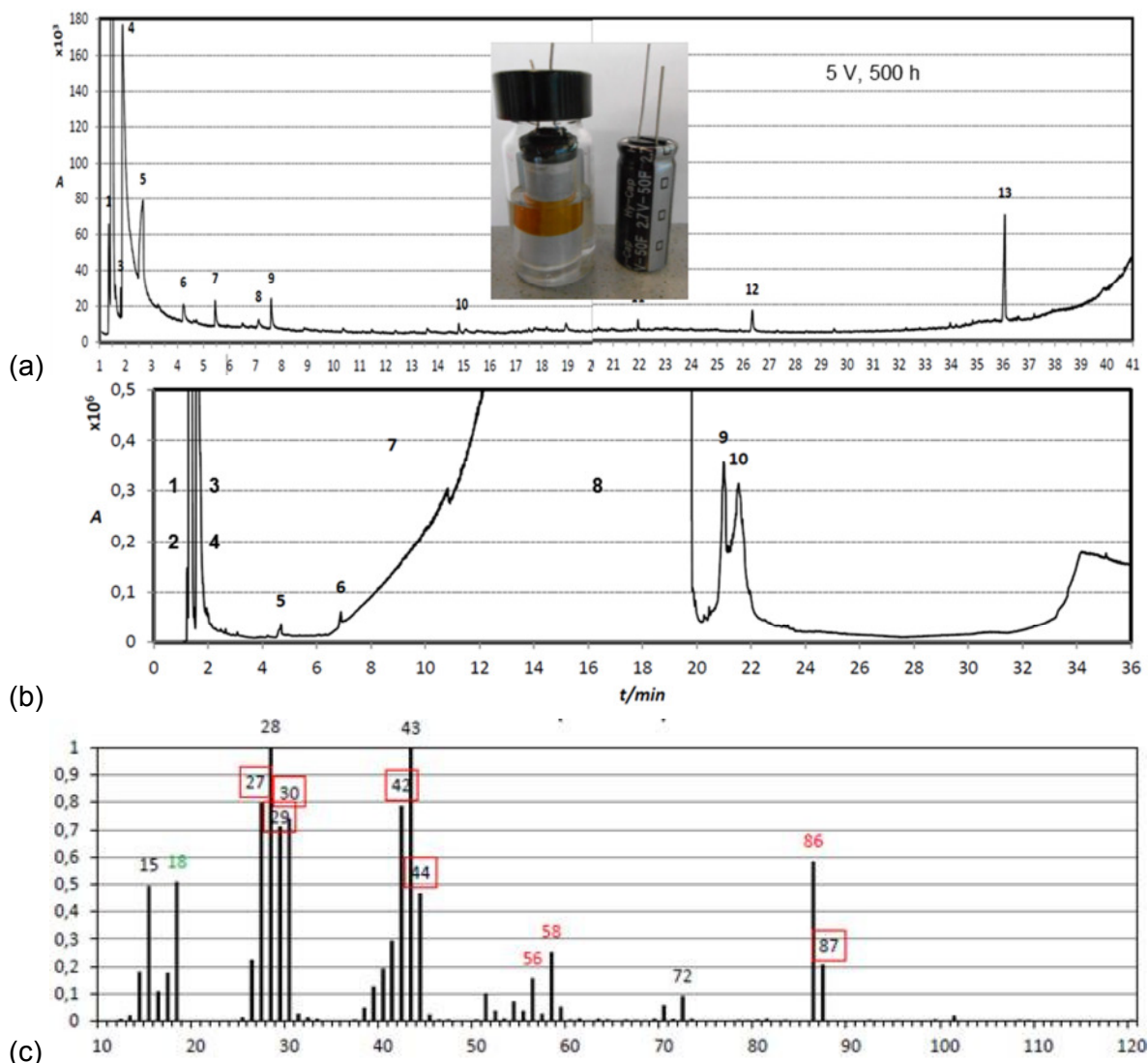
Abbildung 22: Gaschromatogramm der Elektrolytlösung von Aktivkohleelektroden-Separator-Wickeln nach Überspannungsversuchen. Temperaturprogramm: 60... 280 °C, Split 10 : 1. (a) Acetonitril/ \text{Et}_4\text{NBF}_4 nach 5 V für 500 h. 1: 1,1-Difluorethan (!), 2 Acetonitril, 3 Butannitril, 4 Triethylamin, 5 Acetamid ( m/z 59, 44/43/42, 28, 15), 6 N-Ethylacetamid, Hydroxyacetonitril, 7 Diethylamin ( m/z 72/73, 58/59, 44, 28–30), N,N-Diethylformamid ( m/z 101, 86, 72, 58, 42/44, 27–30), Spuren: Propanal, 8 Isocyanatocyclohexan ( m/z 97, 82, 67/69, 54–56, 39–42), 9 N,N-Diethylacetamid ( m/z 115, 72, 58, 42–44, 27, 29/30, 15), 10 Triethylharnstoff ( m/z 144, 100, 72, 56/58, 42/44, 27/29/30), 11 Cyclohexanderivat? N,N-Difluorethanamin? ( m/z 81, 66, 43, 27–29, 15/16) 12 Formamiderivat?, 13 Dicyclohexylharnstoff? ( m/z 224, 143, 98/99, 70, 61, 55/56, 41/43) – (b) Propylencarbonat/ \text{Et}_4\text{NBF}_4 nach 10 V für 7 Tage: 1: 1,1,2-Trifluorethan, 2 Acetonitril (Verunreinigung), 3 Pentylhydroperoxid? 3-Buten-1-ol?, 4 Triethylamin, 5 Methylglyoxal?, 6 Acetanhydrid?, 7 Propan, 8 Propylencarbonat, 9,10 5-Methyloxazolidin? Cyclobutylamin? – (c) Massenspektrum bei Peak 6 (a: 4,32 min) aus ■ N-Ethylacetamid, Hydroxyacetonitril, ■ Triethylamin und ■ Wasser.
