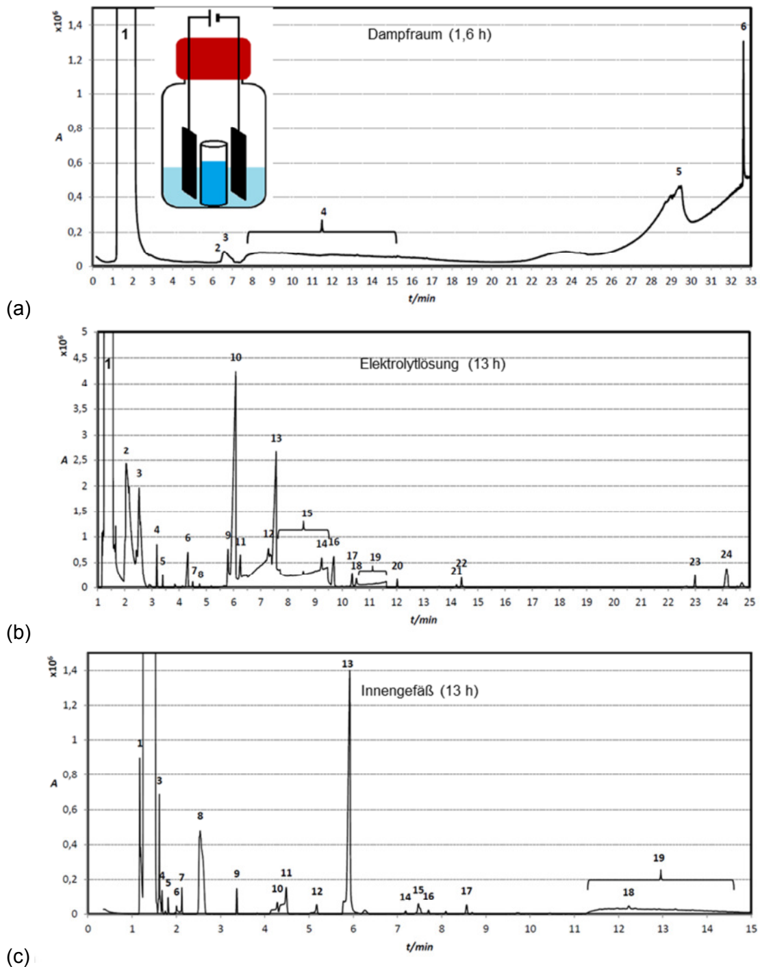
Abbildung 21: Gaschromatogramme während der Elektrolyse von \text{Et}_4\text{NBF}_4 in Acetonitril an Aktivkohleelektroden bei konstantem Strom von 12 \text{ mA cm}^{-2} . (a) Dampfraum: 1 Acetonitril, 2 N -Ethylacetamid, 3 1,4,6-Trimethyl-1,3,5-triazin, 4,5 Triethylamin, 6 Dibutylphthalat. (b) Elektrolyt. (c) Im Acetonitril-Innengefäß absorbierte Stoffe: Substanzen siehe Tabelle 4.
