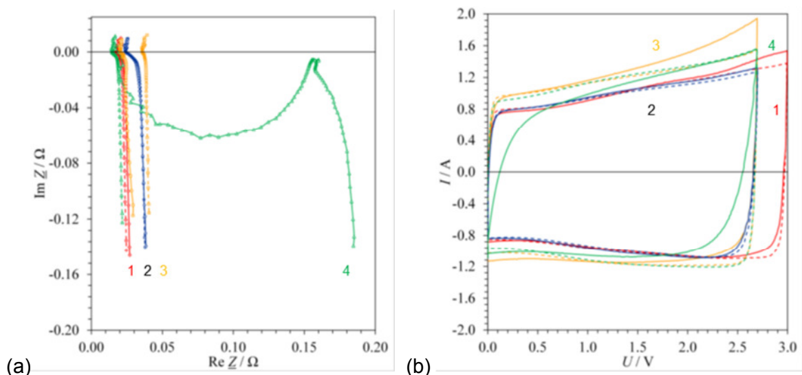
Abbildung 25: Thermische Beständigkeit von 50-F-Superkondensatoren unterschiedlicher Technologie (--- neu, — gealtert, bis 120 °C über 144 h). 1: Vina 3,0 V (Aktivkohle, Acetonitril), 2: Heter-Lampson 2,7 V (Propylencarbonat), 3: SPSCAP 2,7 V, 4: PowerStor 2,7 V, 60 F (Aerogel). (a) Impedanzspektrum, (b) voltametrische Lade-Entlade-Kurve.
