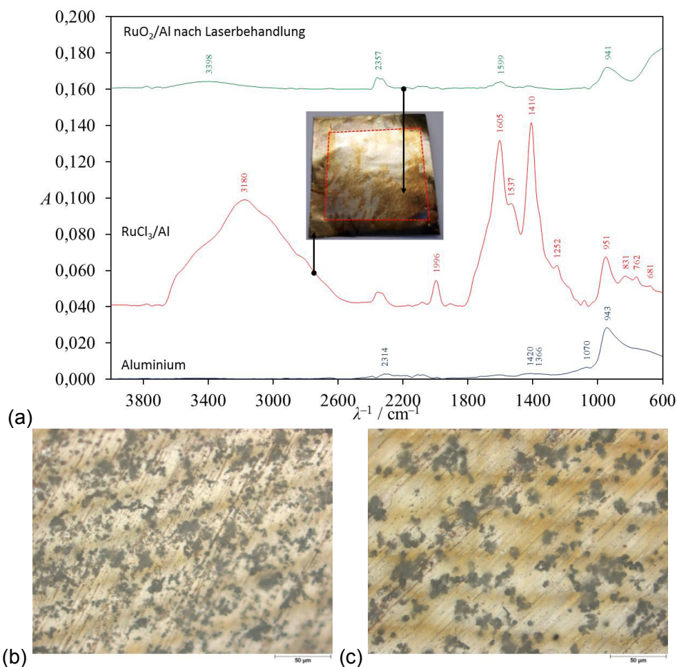
Abbildung 14: (a) Infrarotspektroskopischer Nachweis der unvollständigen Laserthermolyse von wasserhaltigem Rutheniumtrichlorid zu Rutheniumdioxid. Rot: bearbeitete Fläche ( 33 \text{ mm} \times 33 \text{ mm} ). (b) Inhomogene \text{RuCl}_3 -Inseln auf Aluminium nach der Beschichtung aus Aceton und (c) Isopropanol.
