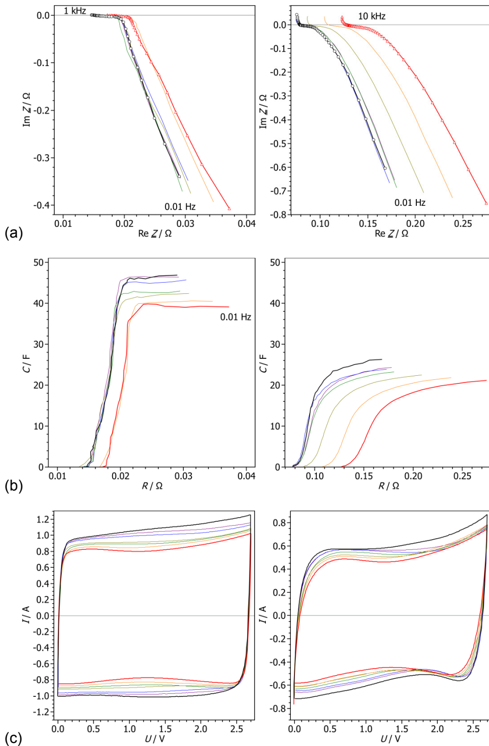
Abbildung 26: Thermische Alterung eines 50-F/2.7-V-Superkondensators (60 °C bis 120 °C, 144 h: schwarz → rot). Links: neues Bauteil, rechts: gebrauchtes Bauteil aus einem mehrjährigen Langzeit-Zyklentest. (a) Impedanzspektren in mathematischer Konvention. (b) Frequenzgang von Innenwiderstand R = \text{Re } \underline{Z} und Kapazität C = [2\pi f \text{Im } \underline{Z}]^{-1} . (c) Voltammetrische Lade-Entlade-Kurve.
