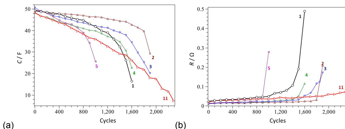
Abbildung 28. Beschleunigter Lade-Entlade-Alterungstest von 50-F-Superkondensatoren durch Zyklisierung bei 3.7 V, 7 A für 30 s. (a) Verlust der Kapazität und (b) Anwachsen des Innenwiderstands. 1 Nesscap, 2 Vina, 3 Vitzrocell, 4 Samwha, 5 Yec, 11 Heter-Lampson.
