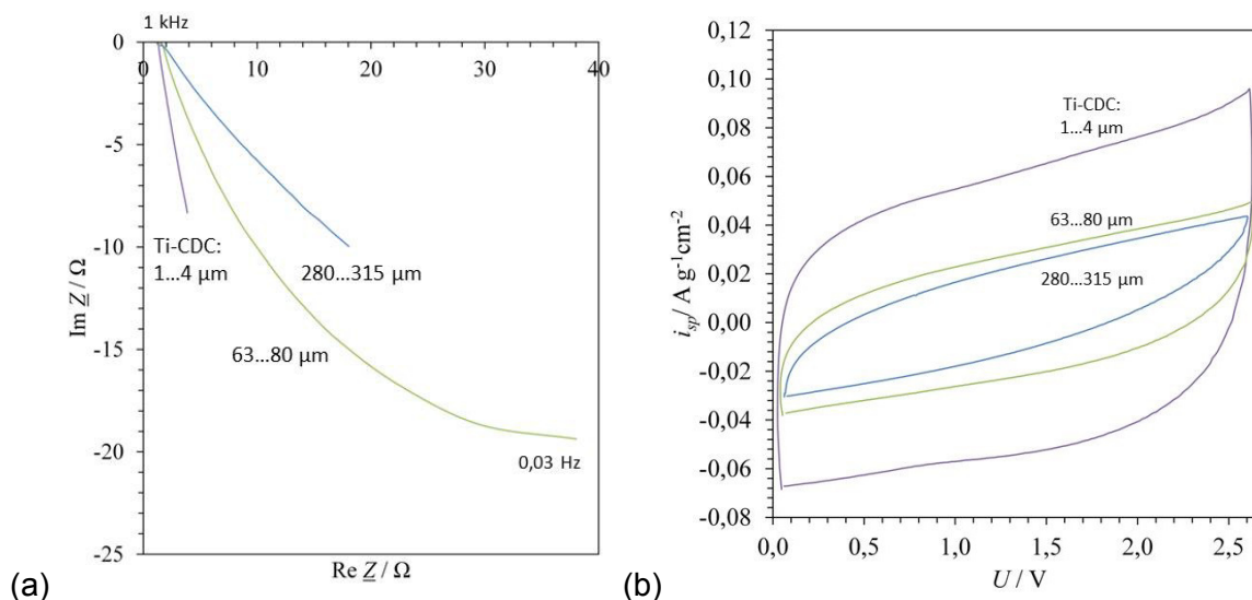
Abbildung 5: Ti-CDC-Elektroden unterschiedlicher Partikelgröße in 1 mol L -1 Et 4 NBF 4 in Acetonitril: (a) Impedanzspektrum, (b) Cyclovoltogramm, normiert auf Aktivmasse und Querschnittsfläche, 50 mV s -1 , IR -Drop korrigiert.
