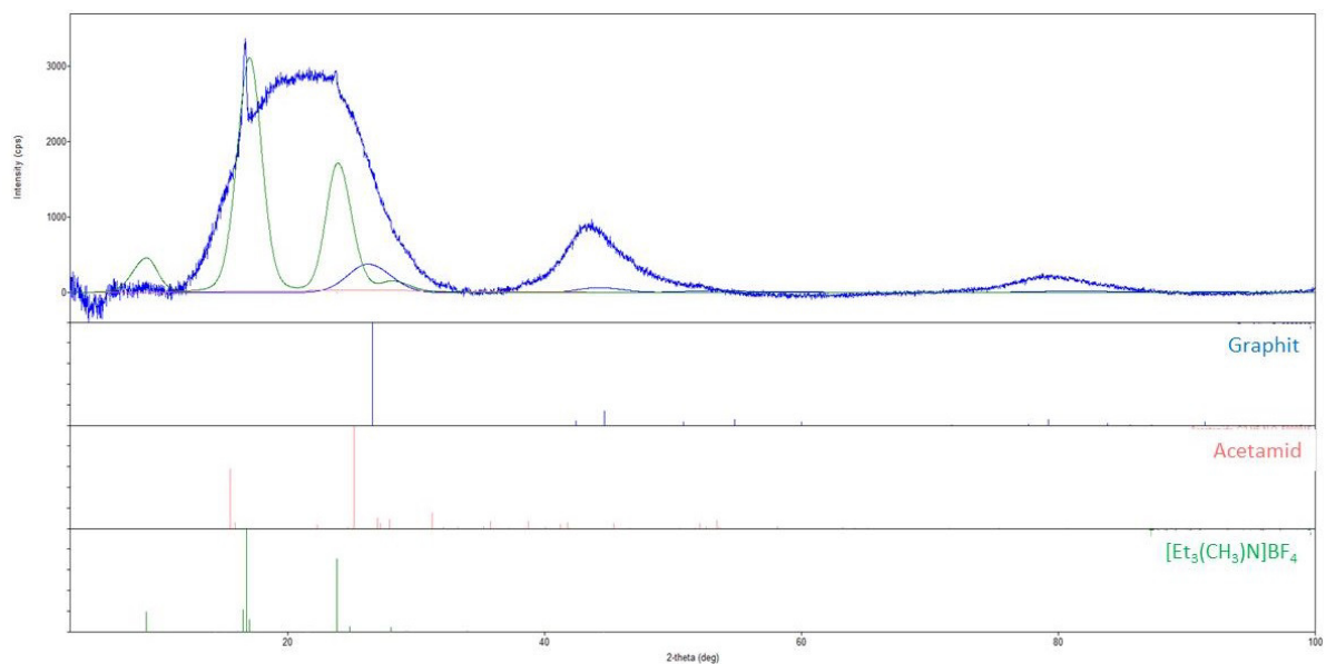
Abbildung 29. XRD-Spektrum einer Kohlenstoffelektrode aus einem thermisch gealterten Superkondensator (Skeleton, 2,85 V, 350 F) mit Rückständen des Leitsalzes und dem Alterungsprodukt Acetamid.
