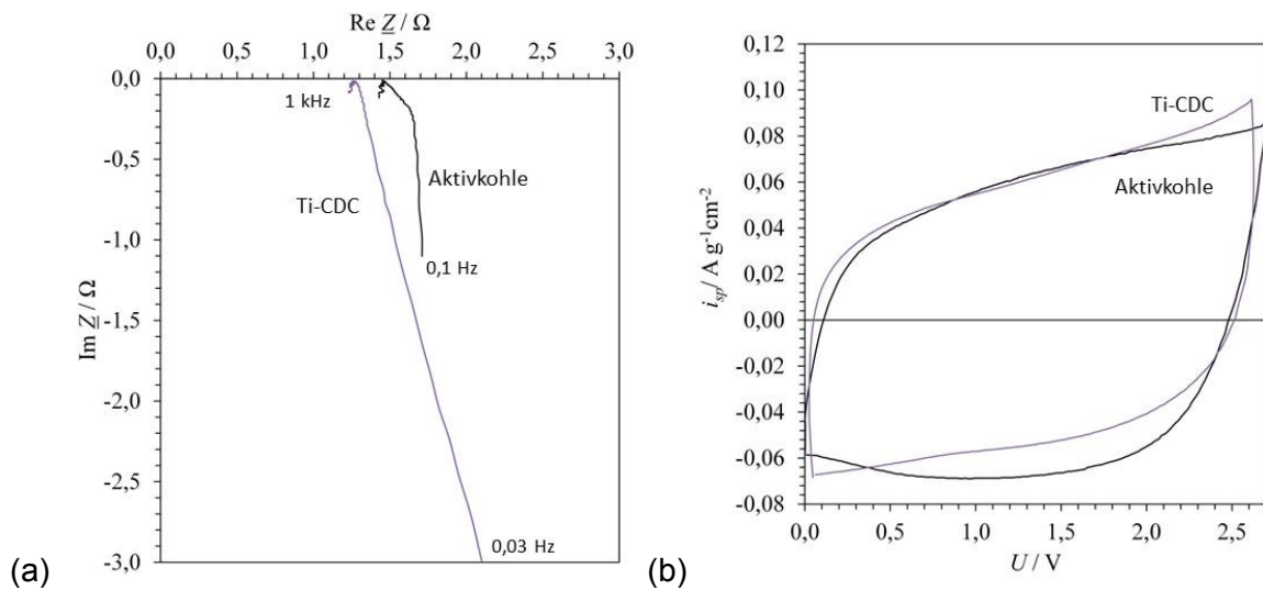
Abbildung 6: Zelle aus zwei gleichen Ti-CDC-Elektroden (Partikelgröße 1-4 \mu\text{m} , 5 % Leitruß Vulcan XC72R, 2 % Na-CMC, 3 % SBR-Binder) in 1 mol \text{L}^{-1} \text{Et}_4\text{NBF}_4 in Acetonitril im Vergleich zu kommerziellen Aktivkohleelektroden: (a) Impedanzspektrum, (b) Cyclovoltogramm, normiert auf Aktivmasse und Querschnittsfläche 12,5 \text{ cm}^2 , 50 \text{ mV s}^{-1} , IR -Drop korrigiert.
