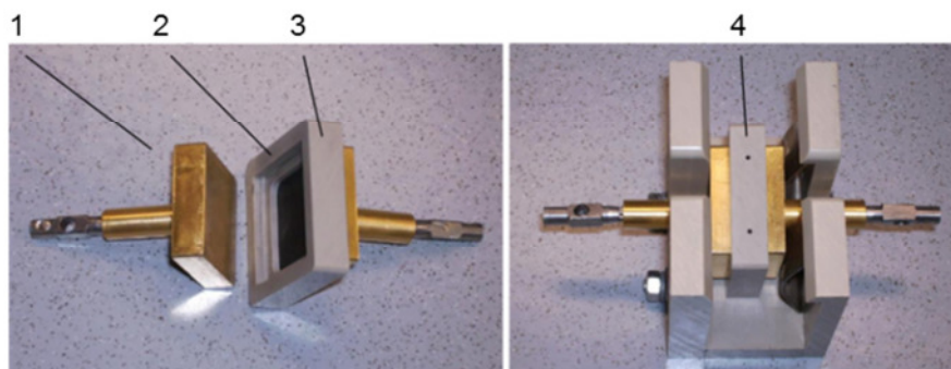
Abbildung 2: Zweielektrodenanordnung 16 mit vergoldeten Kupferstempeln 1 (9 cm 2 ), Dichtung 2 , Rahmen 3 und Einfülllöchern für den Elektrolyten 4 .
