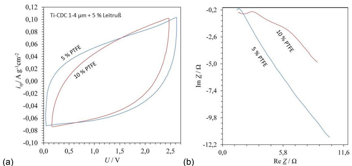
Abbildung 3: Ti-CDC-Elektroden von 1 bis 4 µm Partikelgröße mit Rußzusatz und 5 % bzw. 10 % Fluorpolymer-Binder. (a) voltammetrische Lade-Entlade-Kurve in 1 \text{ mol L}^{-1} \text{ Et}_4\text{NBF}_4 in Acetonitril. (b) Impedanzspektrum.
