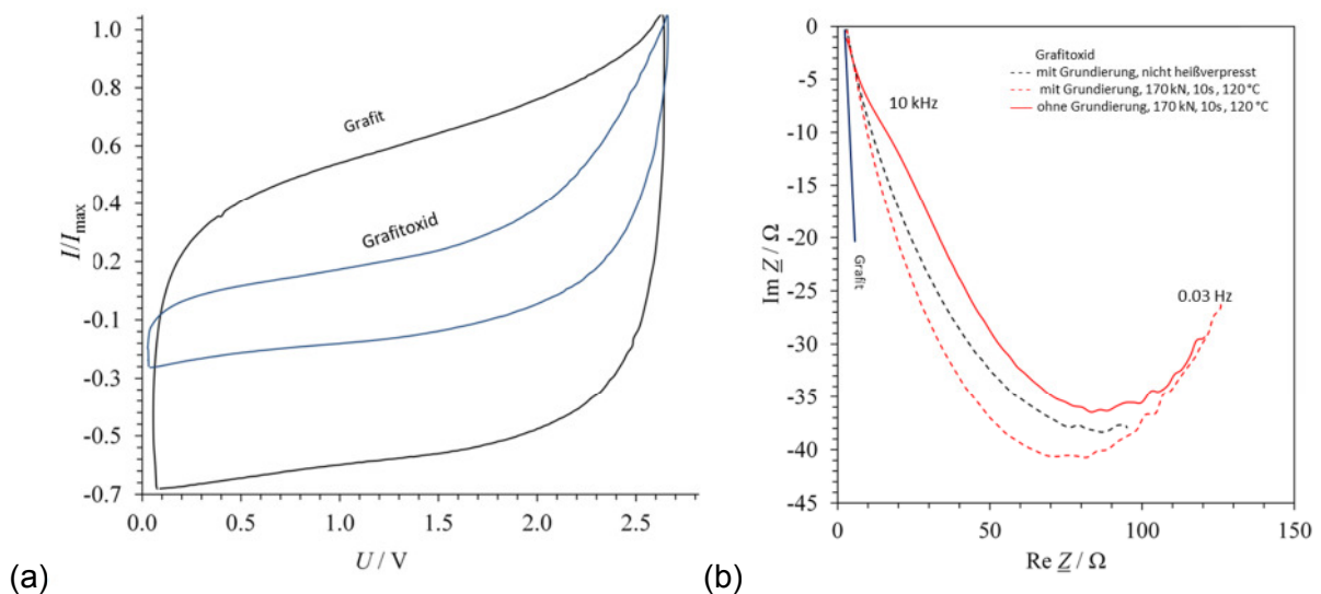
Abbildung 10: (a) Voltammetrische Strom-Spannungskurven von kautschukgebundenem Reinflockengrafit und Grafitoxid auf Aluminiumträger, auf den größten Strom bezogen. Zweielektroden-Anordnung, 50 mV/s, 1 M Et 4 NBF 4 in Acetonitril, IR -Drop korrigiert, Elektrodenquerschnitt 6,25 cm 2 . (b) Impedanzspektren: Grafitoxid (90 % Grafitoxid, 5 % Ruß C65, 3 % SBR, 2 % NaCMC) mit und ohne Heißverpressung.
