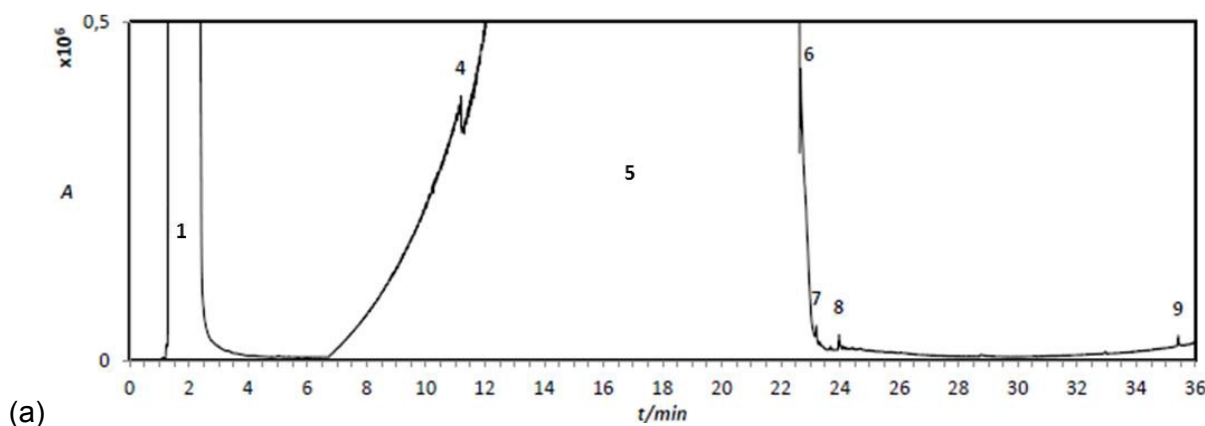
Abbildung 23: Gaschromatogramm der Elektrolyse von 1 mol/L \text{Et}_4\text{NBF}_4 in Propylencarbonat, 60–280 °C, Split 10 : 1: Gasraum nach 4,5 V (7 d): 1 Acetonitril (60 °C), 4/6 Propan 70–90 °C), 5 Propylencarbonat, 7 Essigsäureanhydrid? (150 °C, m/z 43), 8 Propanaminderivat (150 °C), 9 Carbonsäureester (224 °C).
